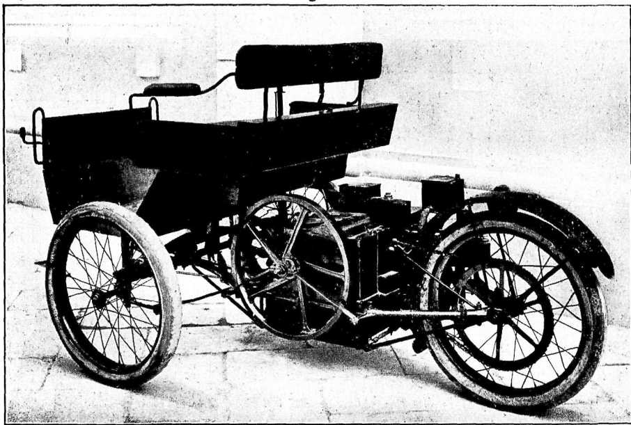
LX - ALLA MOSTRA DEI MOTORI A SCOPPIO NELLA FIERA CAMPIONARIA VETTURETTA TRICICLO BERNARDI HP 1,5 - 2 - 5 - 1894
