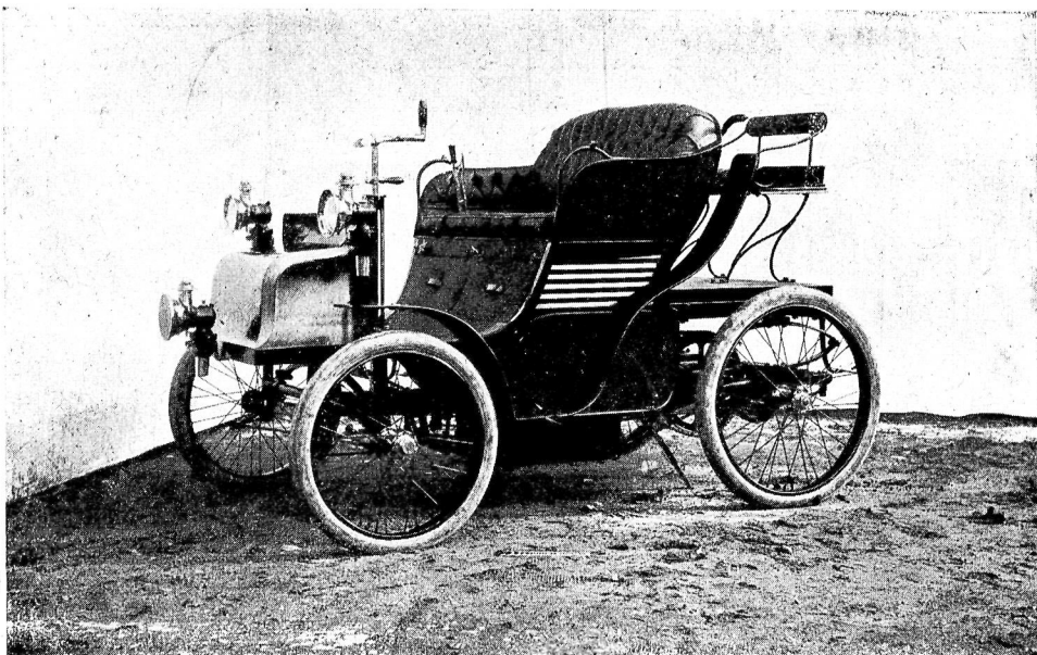
LXI - ALLA MOSTRA DEI MOTORI A SCOPPIO NELLA FIERA CAMPIONARIA - SPIDER BERNARDI - H-P 2,5
